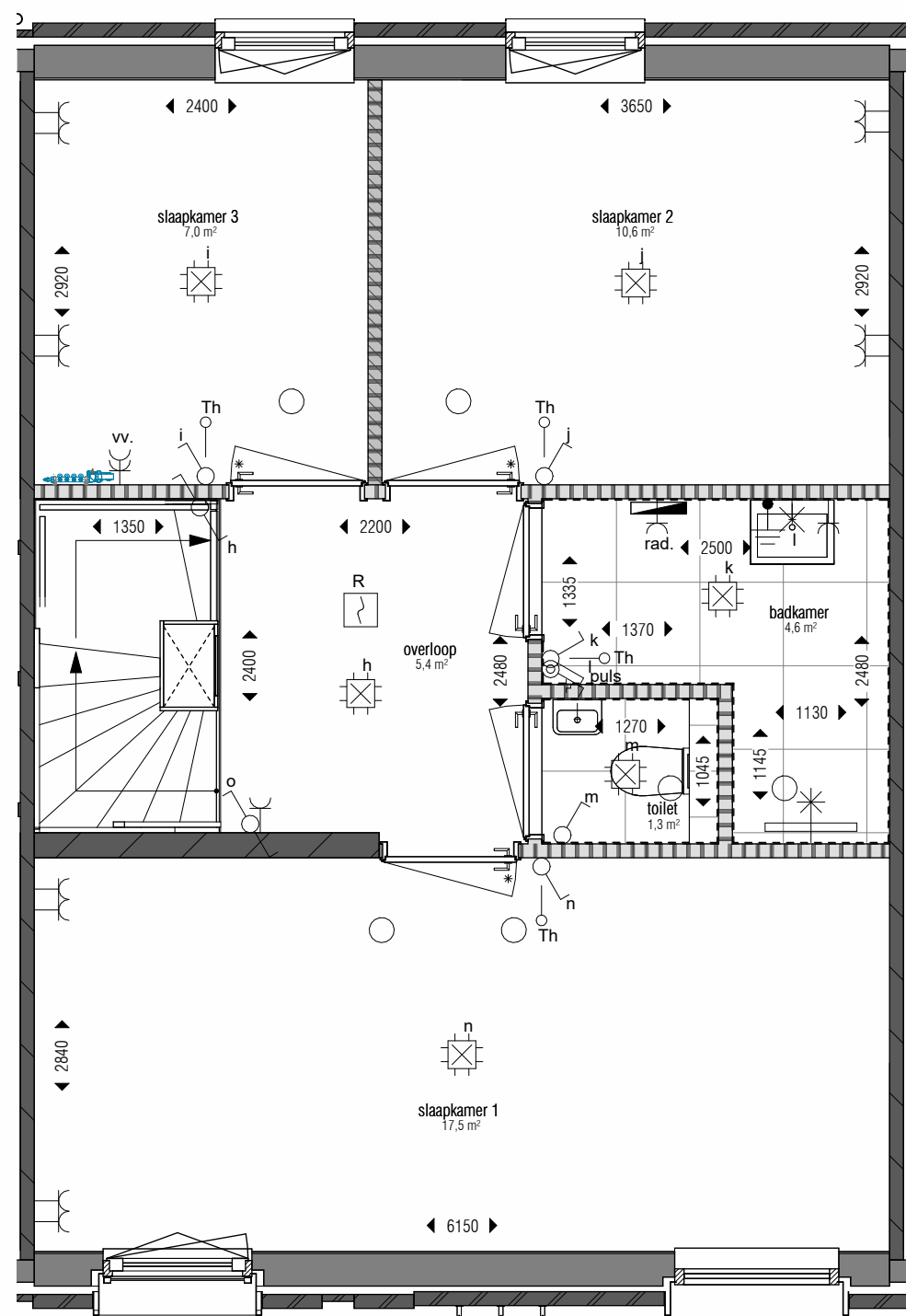
eerste verdieping 1 : 50
