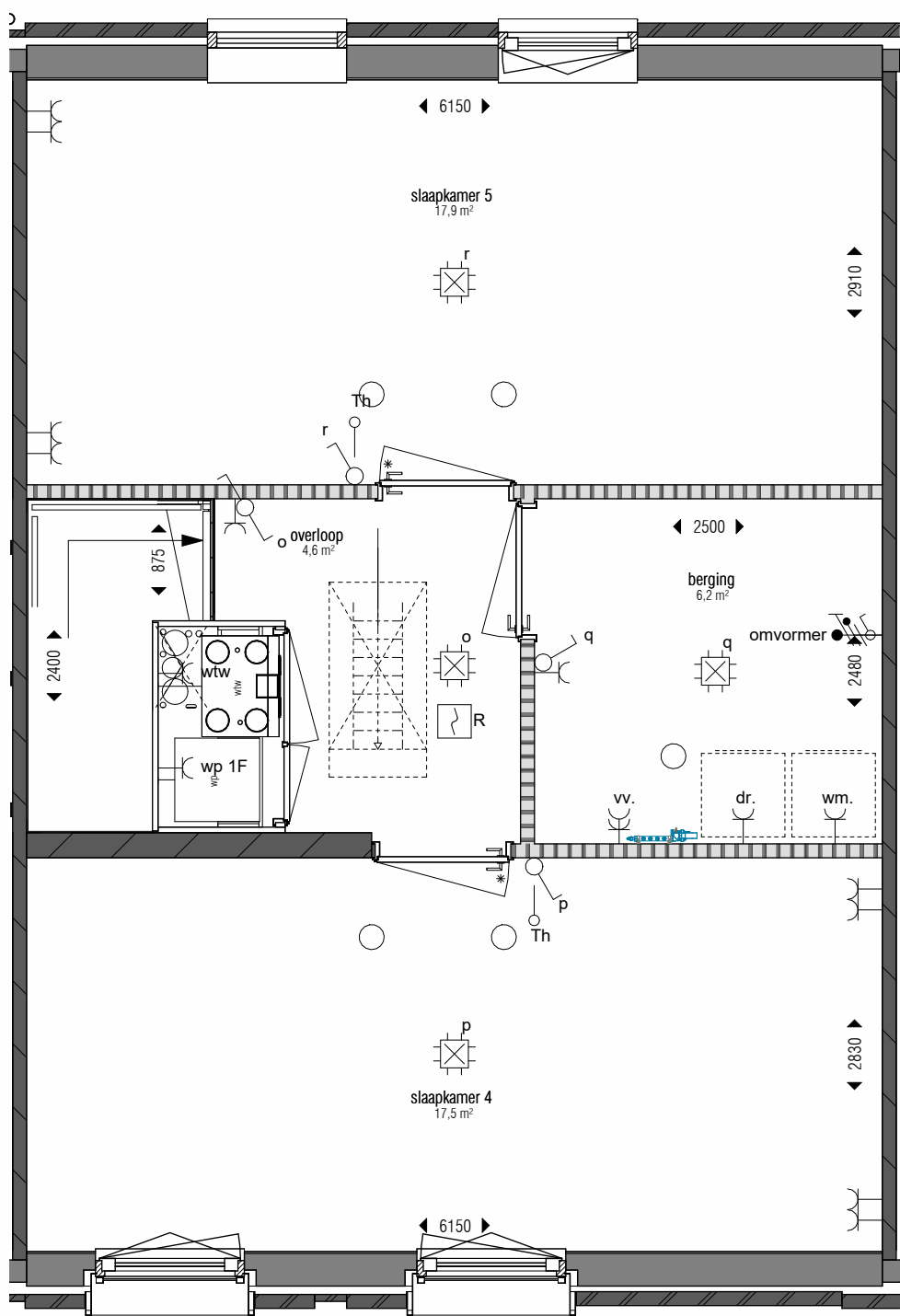
tweede verdieping 1 : 50
