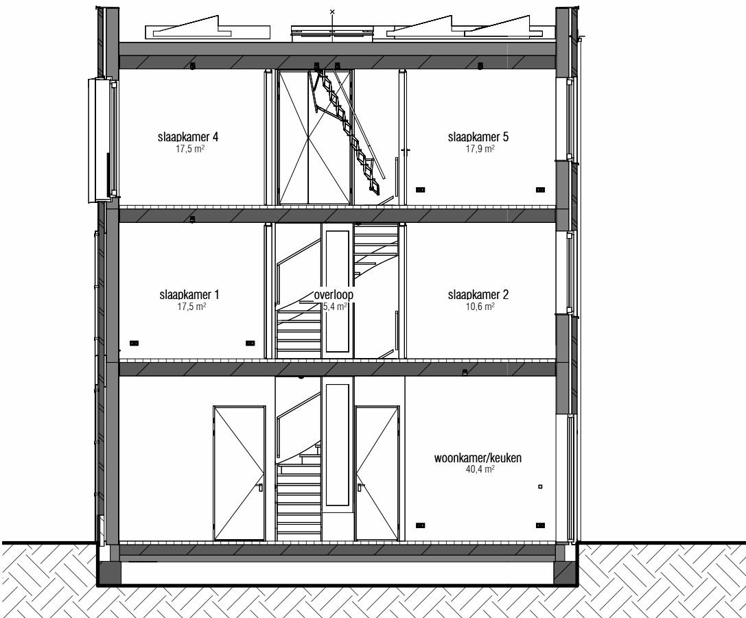
doorsnede 1 : 100
