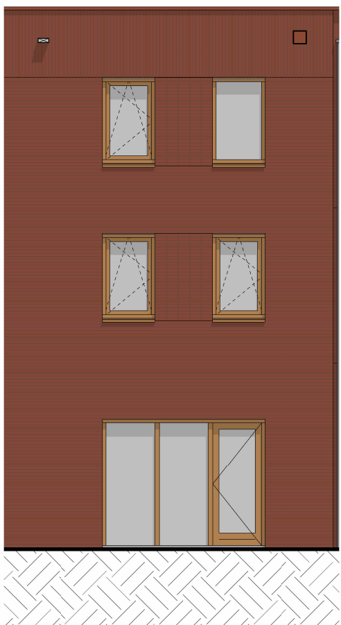
achtergevel 1 : 100
