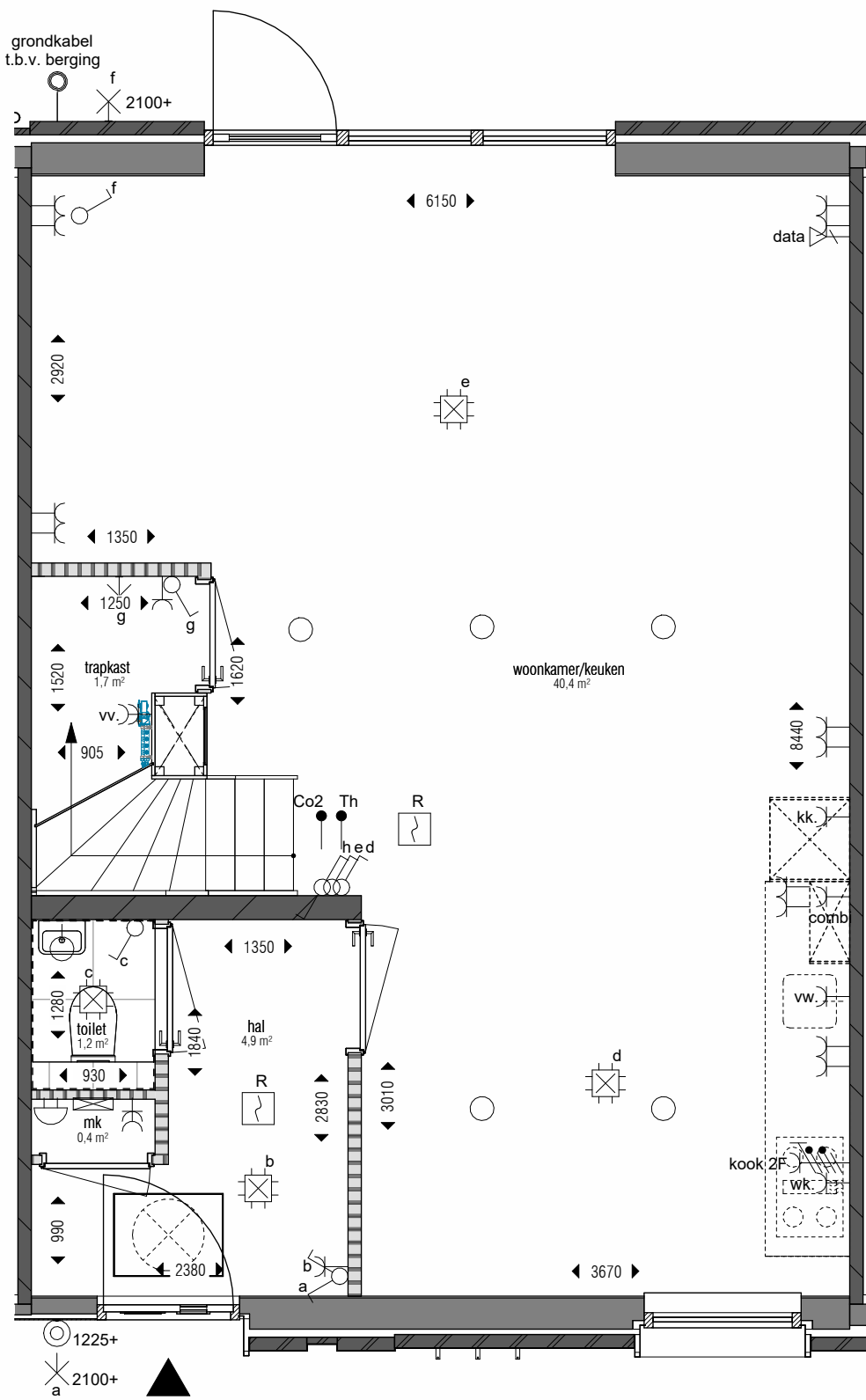
begane grond 1 : 50
